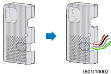
Afbeelding6-8 Kabels uit de kabelopening leiden
