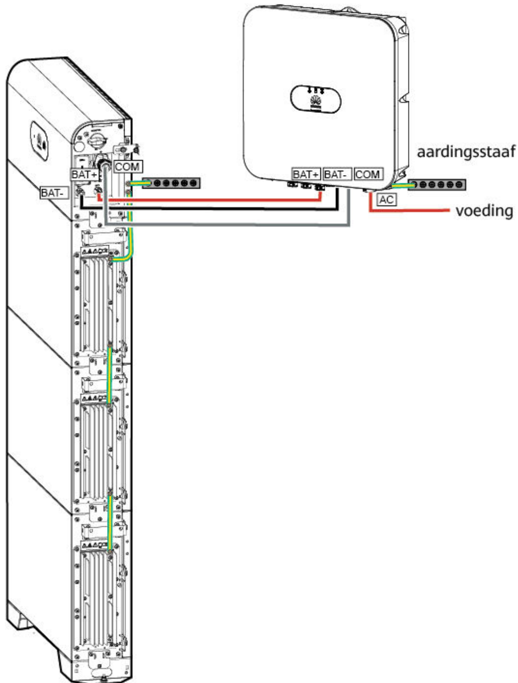
Afbeelding8-3 Kabelaansluitschema
