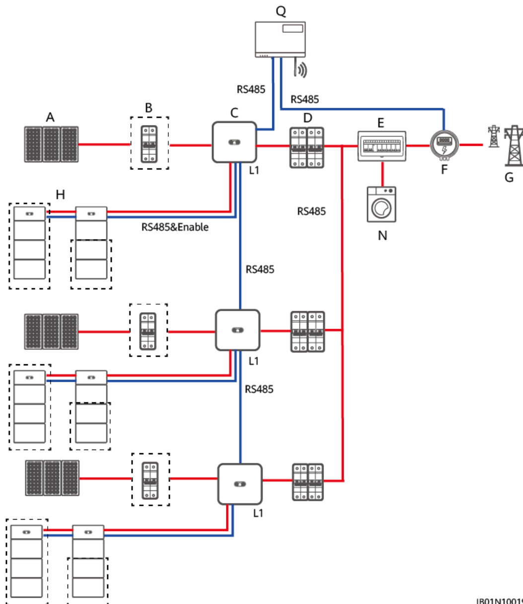
Afbeelding4-3 Netwerkdigram van SUN2000-(2KTL-6KTL)-L1-omvormers in cascade (kaders met stippellijn geven optionele componenten aan)
