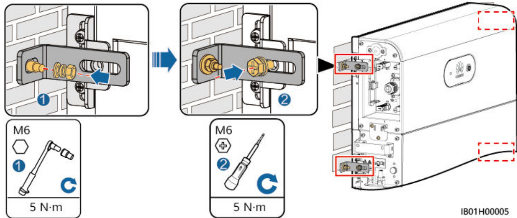
Afbeelding5-9 De vermogensregelmodule vastzetten
