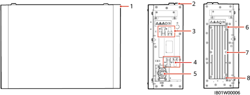
Afbeelding2-8 Batterij-uitbreidingsmodule
