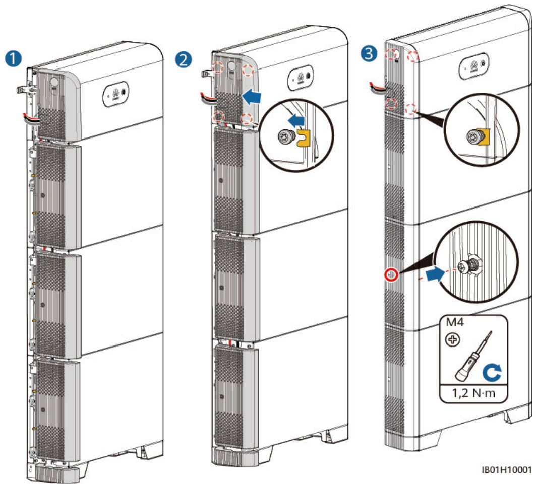
Afbeelding6-19 Kap installeren
