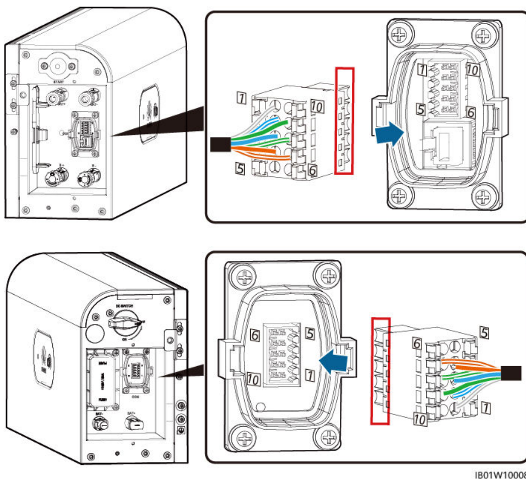
Afbeelding 6-17 De aansluiting plaatsen
