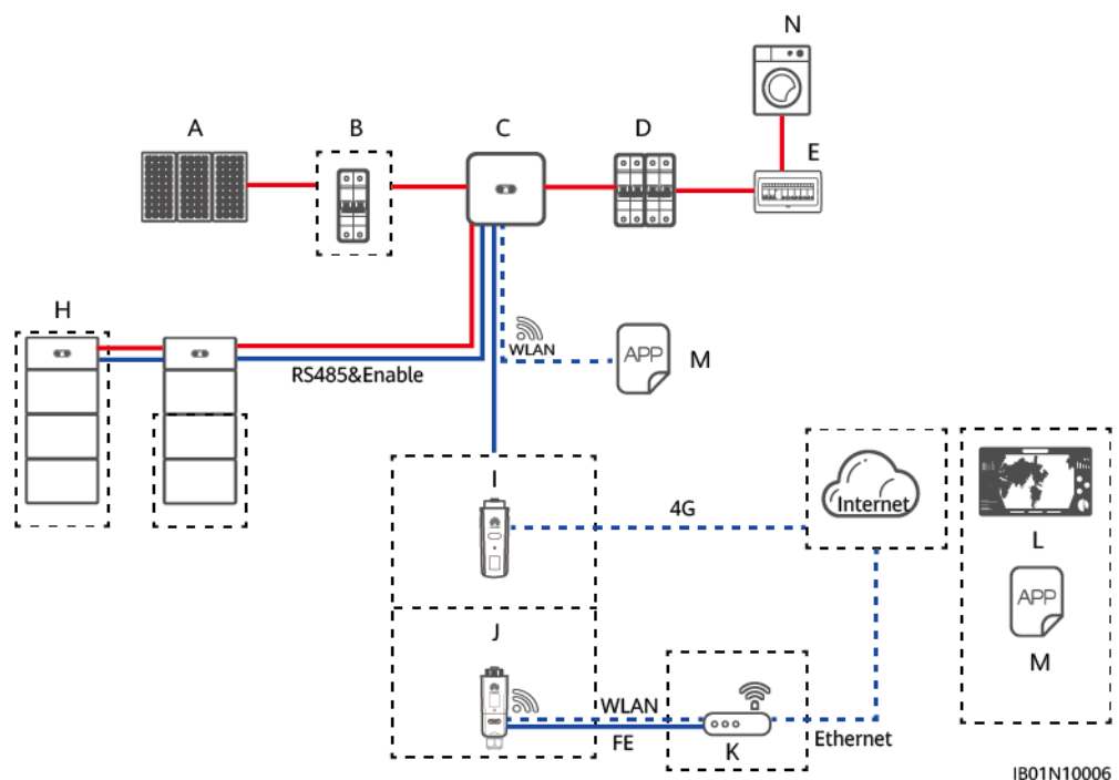
Afbeelding4-16 ESS buiten net (kaders met stippellijn geven optionele onderdelen aan)
