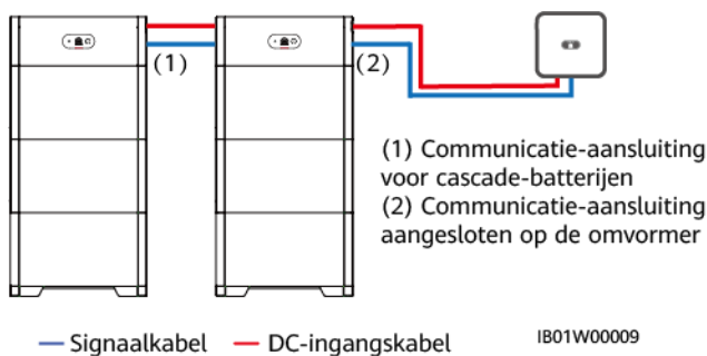
Afbeelding6-16 Cascadekabelverbinding batterij
