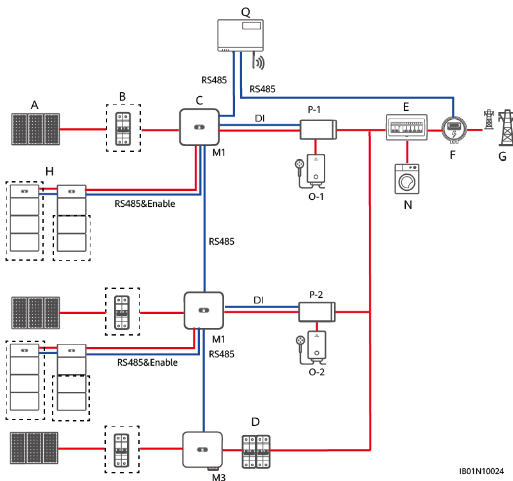
Afbeelding4-12 Netwerk van twee SUN2000-(3KTL-10KTL)-M1-omvormers en één SUN2000-(20KTL, 29.9KTL, 30KTL, 36KTL, 40KTL)-M3-omvormer (kaders met stippellijn geven optionele componenten aan)
