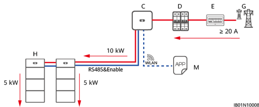
Afbeelding8-1 Netwerkschema voor scenario driefasenvoeding
