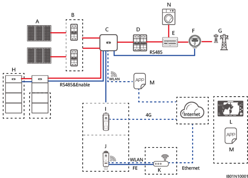
Afbeelding4-1 Netwerkdigram netgekoppeld ESS (kaders met stippellijn geven optionele componenten aan)
