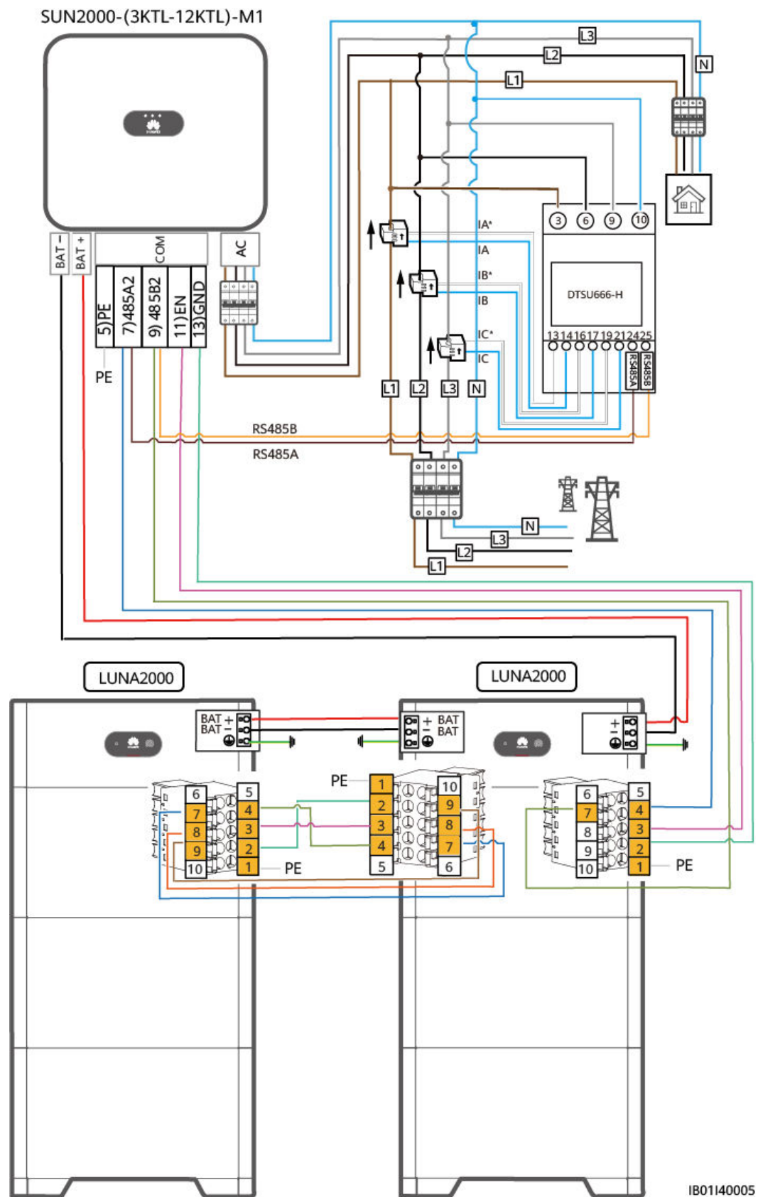
Afbeelding6-7 SUN2000-(3KTL-12KTL)-M1
