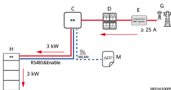
Afbeelding8-2 Netwerkschema voor scenario éénfasevoeding
