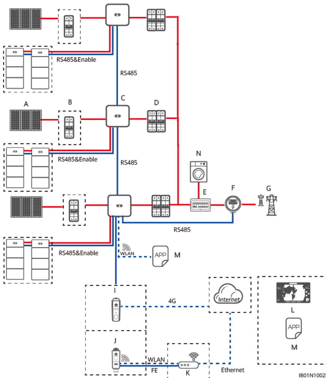
Afbeelding4-4 Smart Dongle-netwerk (kaders met stippellijn geven optionele componenten aan)
