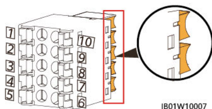
Abbeelding6-13 Signaalkabelpoorten
