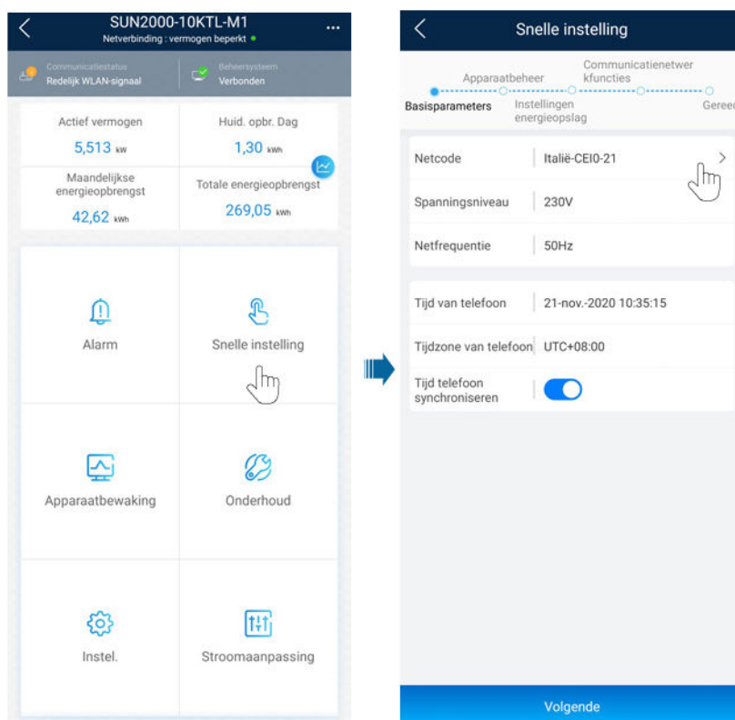
Afbeelding4-17 Instellen van de elektriciteitsnetcode voor buiten het net (Island-Grid)
