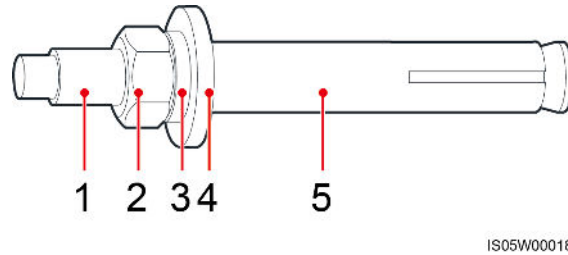
Afbeelding5-3 Structuurschema M6-keilbout
