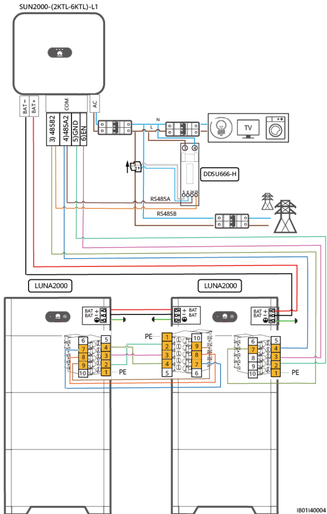
Afbeelding6-6 SUN2000-(2KTL-6KTL)-L1
