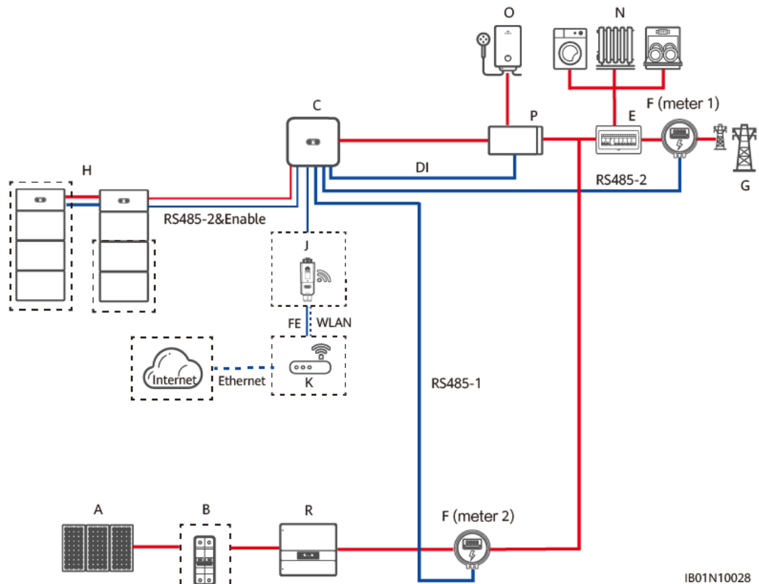
Afbeelding4-18 Netwerk met omvormers van derden
