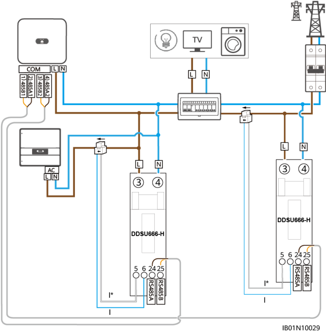
Afbeelding4-19 Kabelaansluitingen stroommeter voor SUN2000-(2KTL-6KTL)-L1
