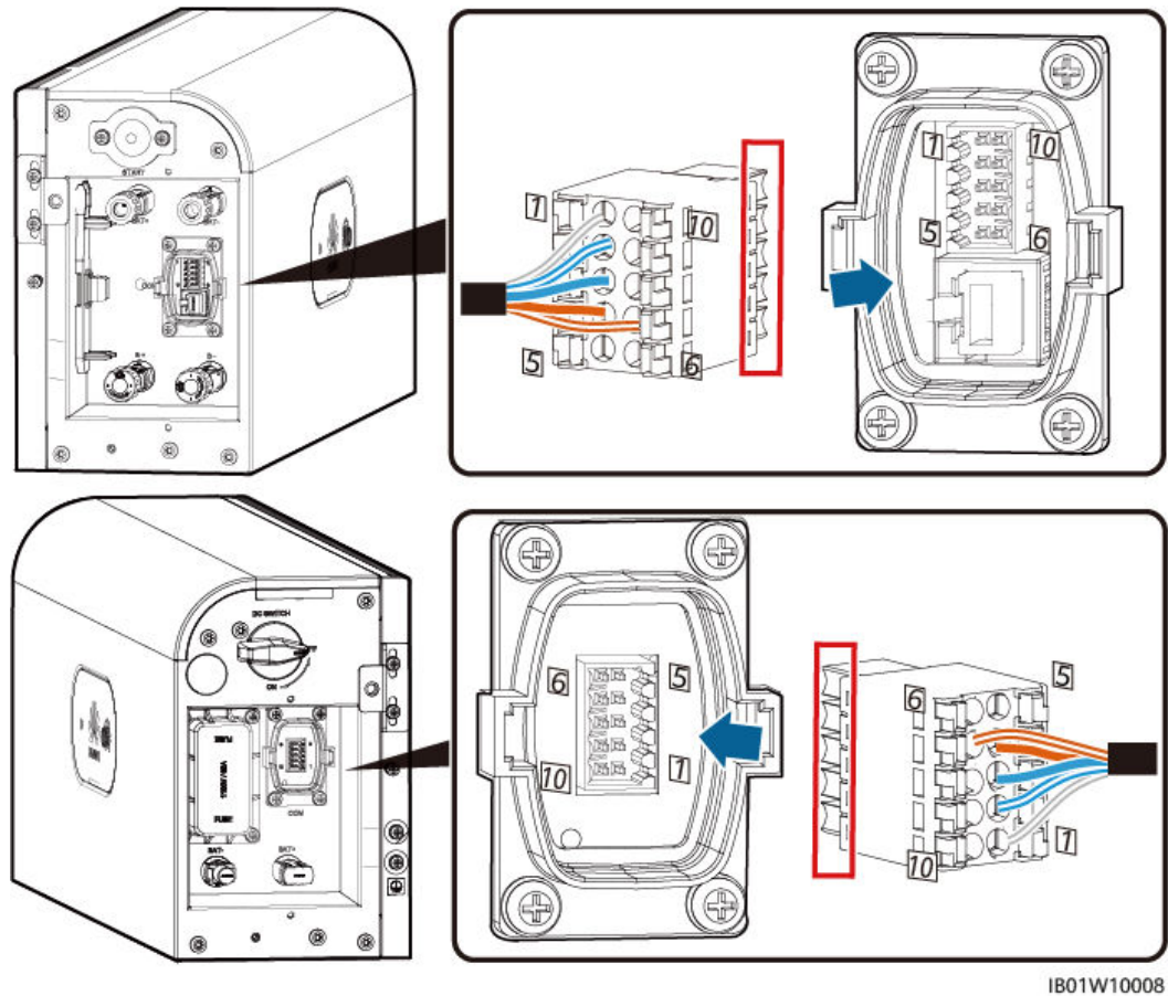
Afbeelding6-14 De aansluiting plaatsen
