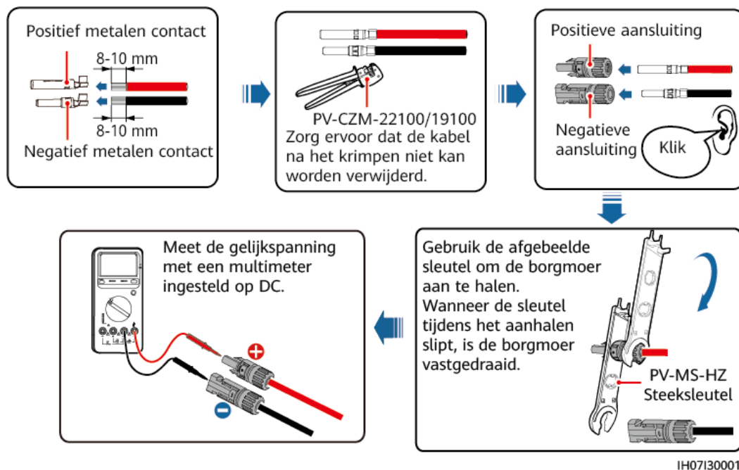
Afbeelding6-11 DC-aansluitingen in elkaar zetten
