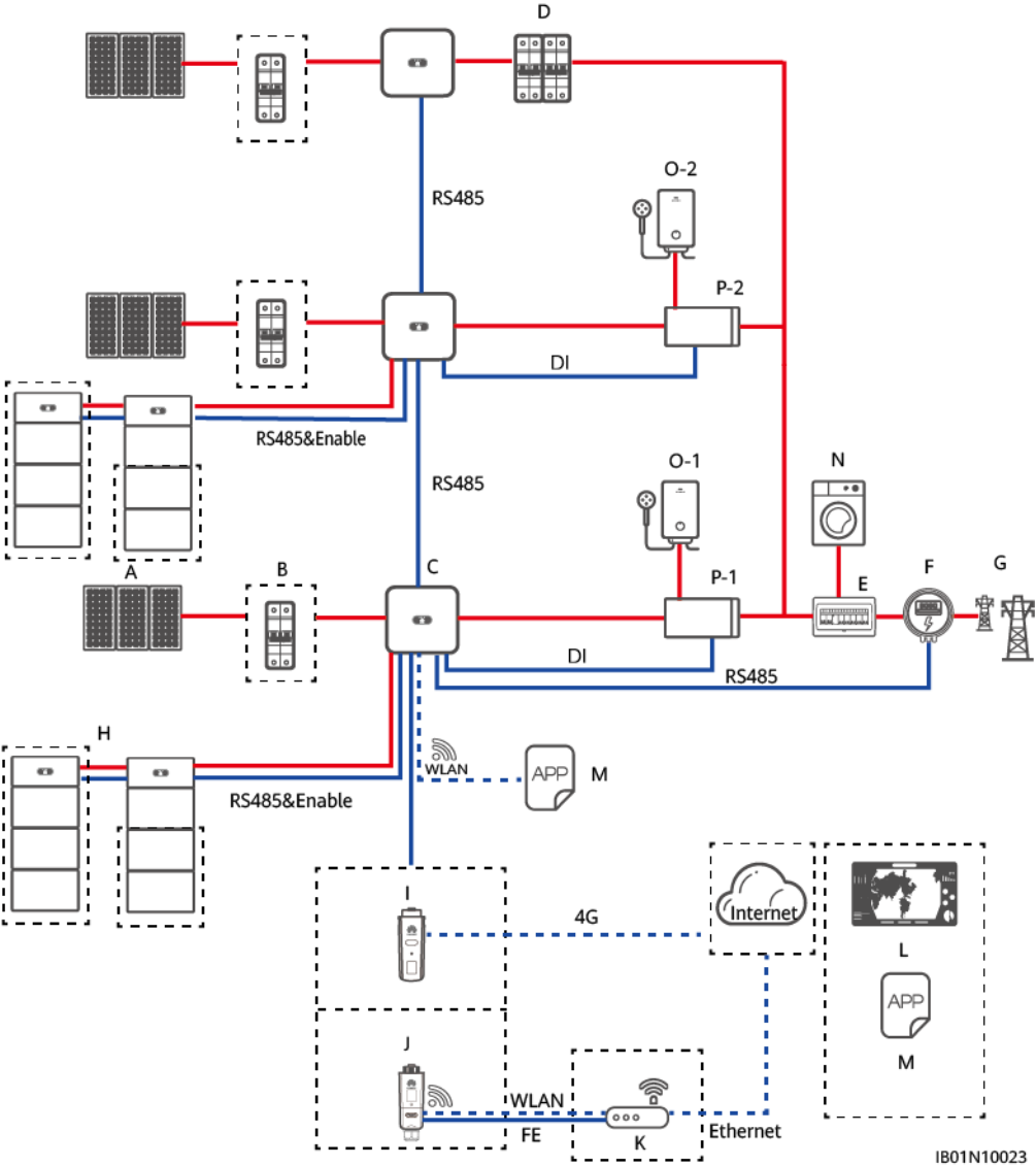
Afbeelding4-14 Smart Dongle-netwerk in een netgekoppeld ESS en ESS buiten net (kaders met stippellijn geven optionele componenten aan)
