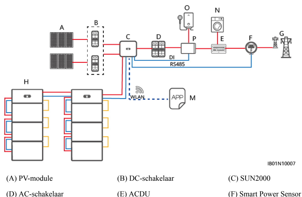
Afbeelding6-1 Batterijkabelverbindingen
