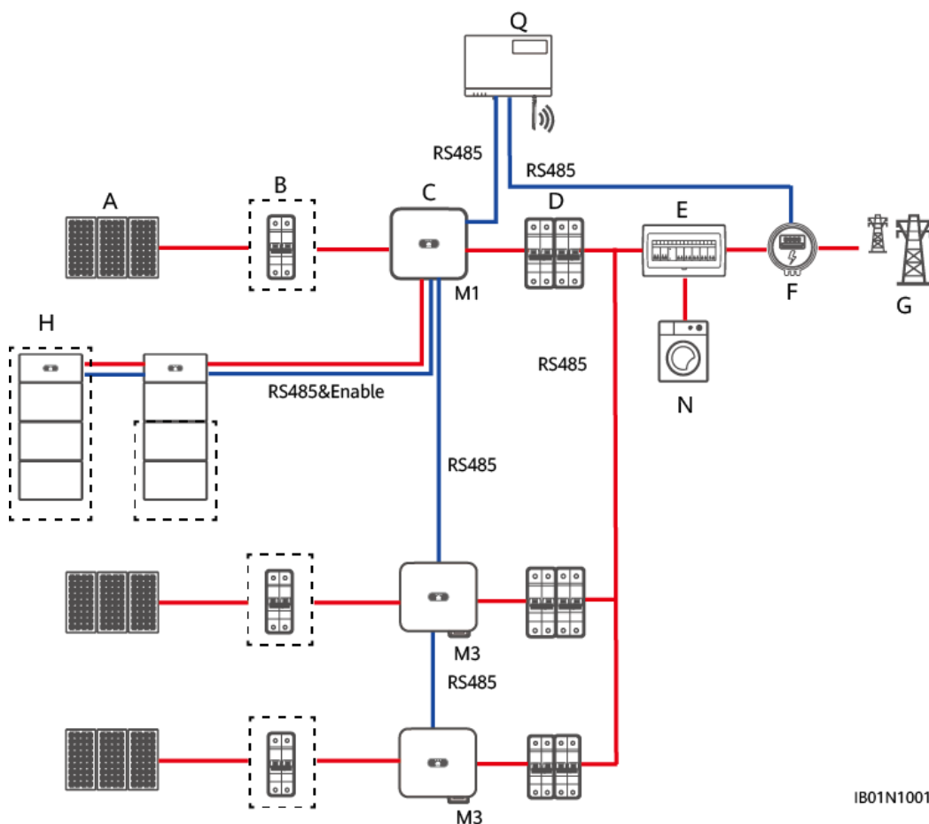
Afbeelding4-2 Netwerk van één SUN2000-(3KTL-10KTL)-M1-omvormer en twee SUN2000-(20KTL, 29.9KTL, 30KTL, 36KTL, 40KTL)-M3-omvormers (kaders met stippellijn geven optionele componenten aan)
