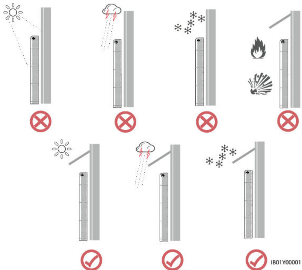
Afbeelding1-3 Installatie-omgeving
