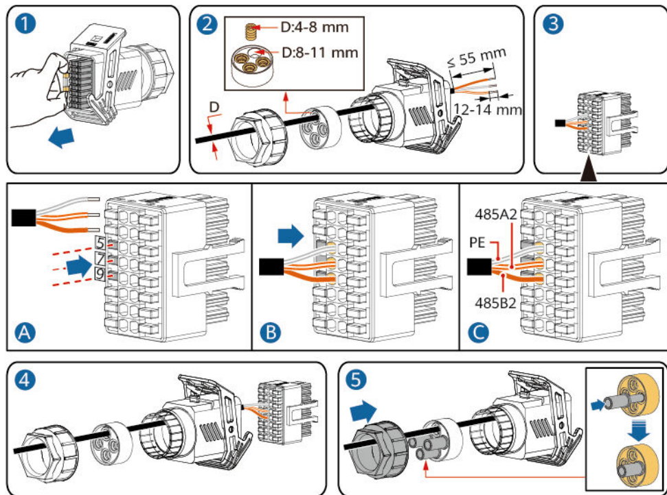
Abbildung 5-30 Kabelmontage
