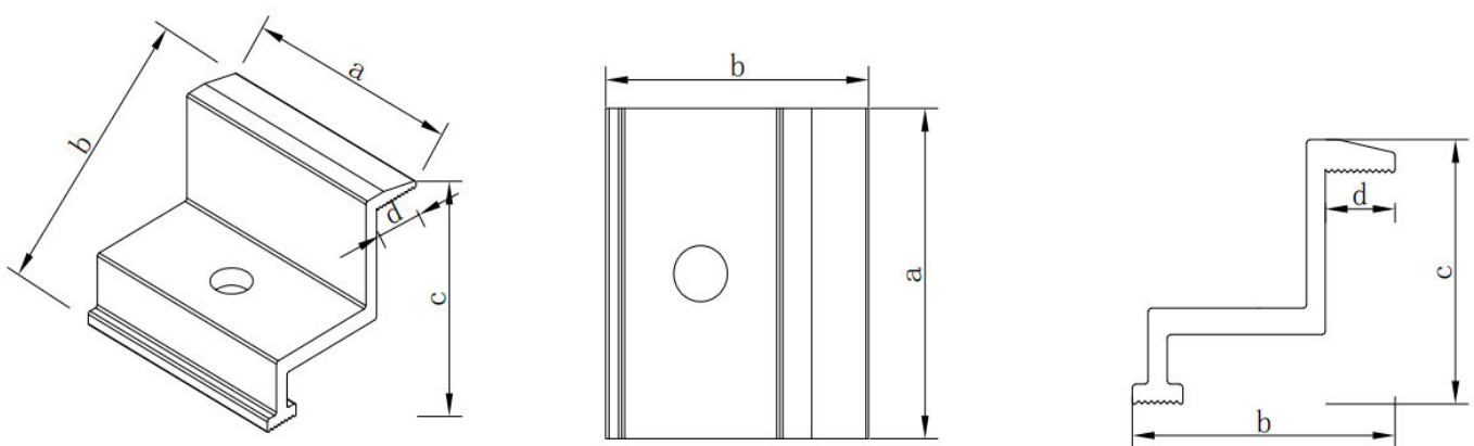
Fig. 5 Clamp
