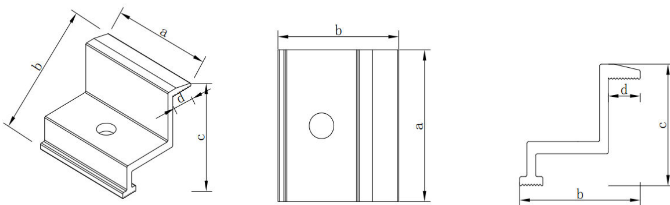
Fig. 5 Clamp
