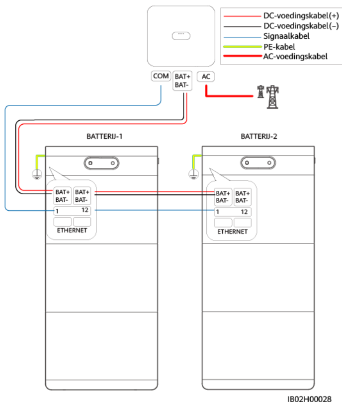
Afbeelding3-1 Kabelaansluitschema
