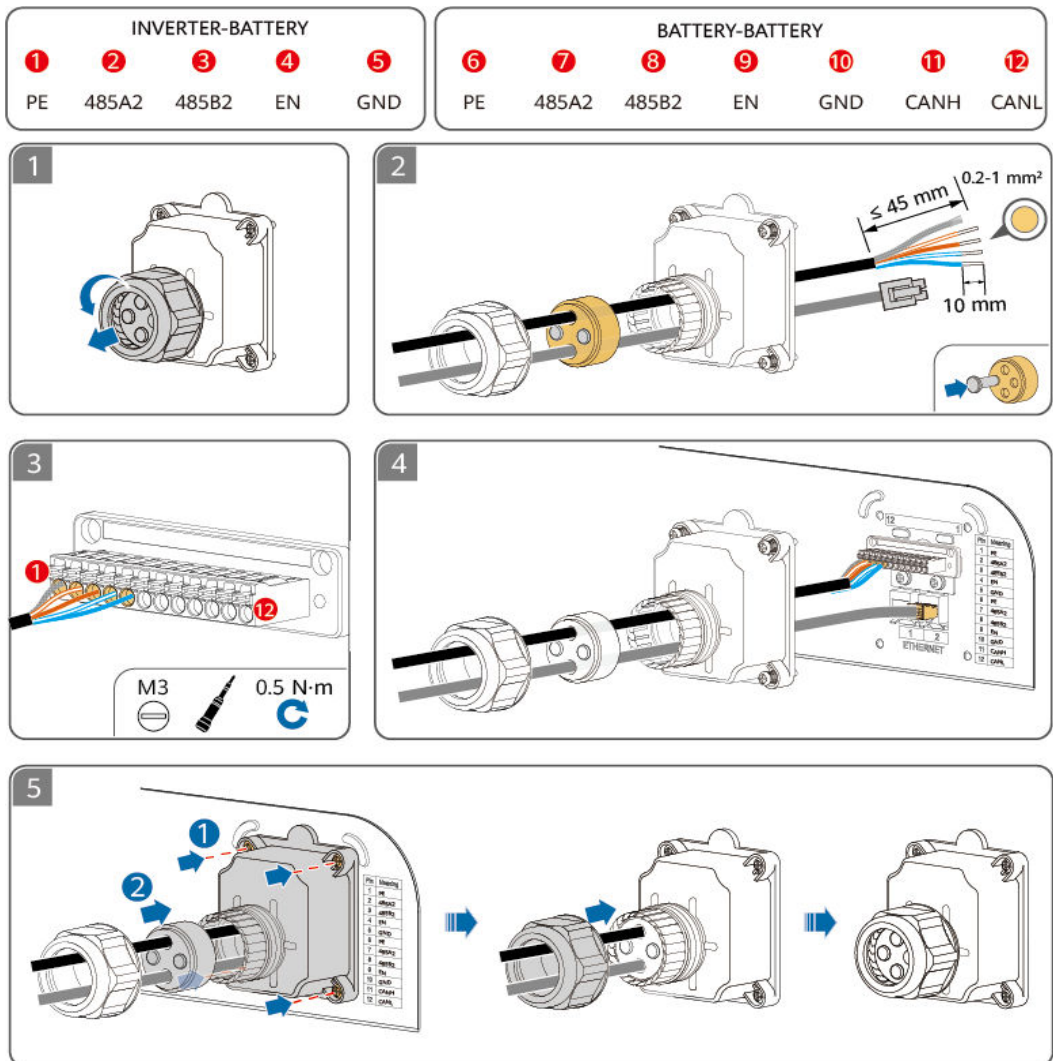
Afbeelding5-7 Signaalpoort aansluitingen
